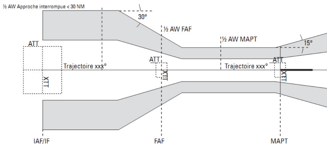
Fig. 3 RNP APCH
