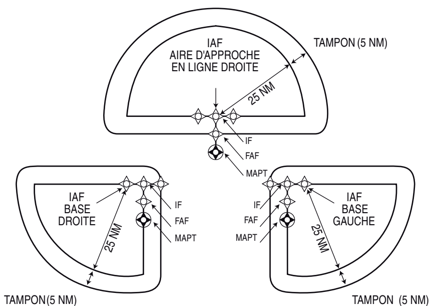
Configuration TAA en T
